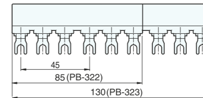
TCMS-32H/HI+PB-32(2,3 Terminal) PB-322(2 Terminal), PB-323(3 Terminal)
