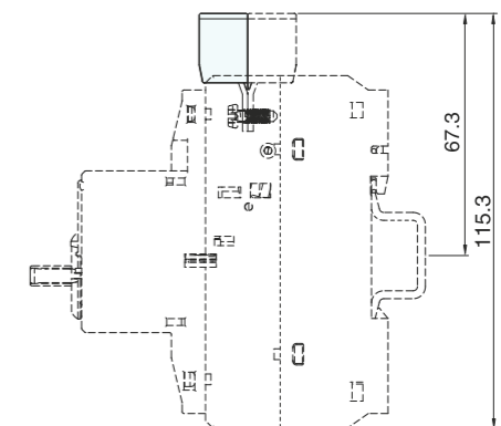
TCMS-32H/HI+PB-32(2,3 Terminal) PB-322(2 Terminal), PB-323(3 Terminal)
